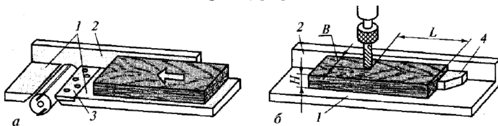
Рис.2. Рухоме а) та нерухоме б) базування заготовок при деревообробці: 1 – стіл, 2 – напрямна лінійка, 3 – накладка, 4 – упор
